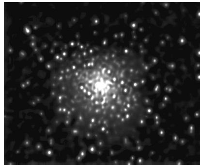
M92 - 5/9/03
