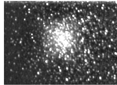
M3 - 4/23/03
