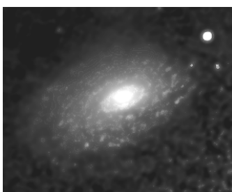
M63 - 4/23/03
