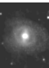
M95 - 4/23/03
