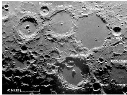
MOON - 8/19/03
