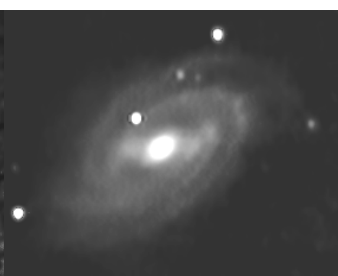
M109 - 4/23/03
