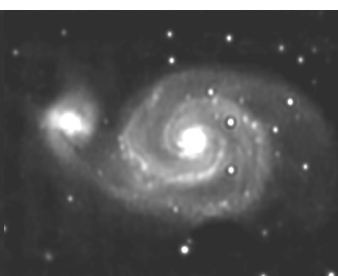
M51 - 4/23/03
