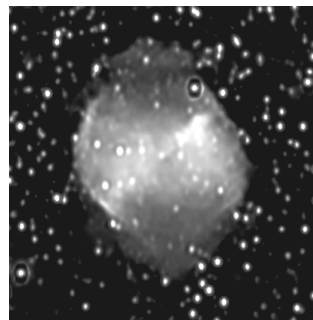
M27 - 5/21/03
