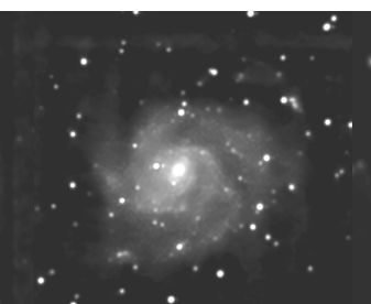
M101 - 4/23/03
