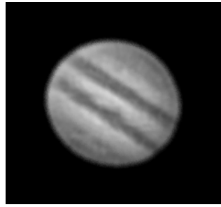
JUPITER - 4/23/03
