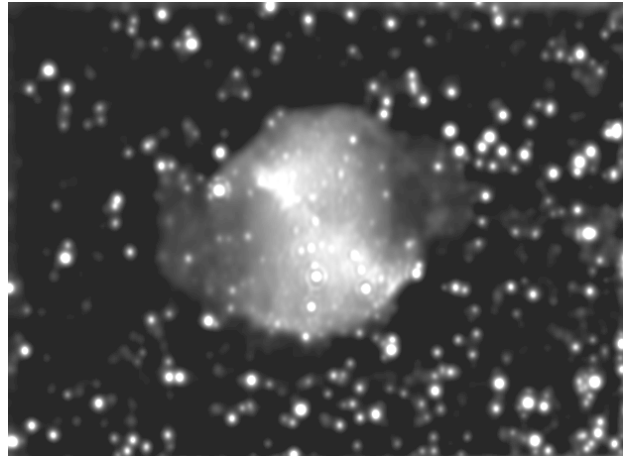
M27 -- Dumbbell Nebula
