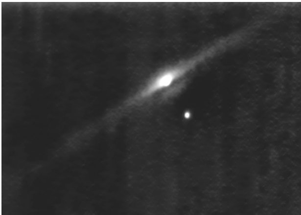
C38 - Edge on Galaxy
